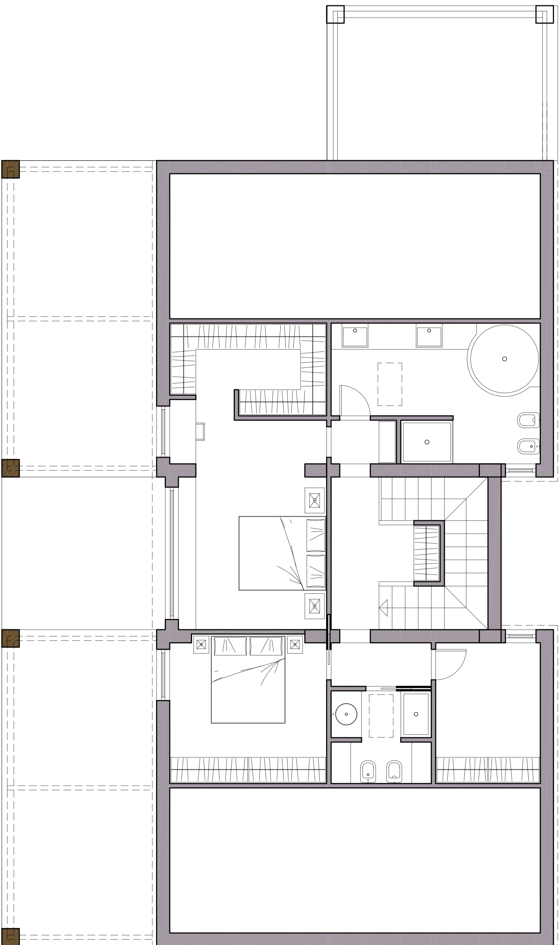
PIANTA PIANO SOTTOTETTO - scala 1:50
