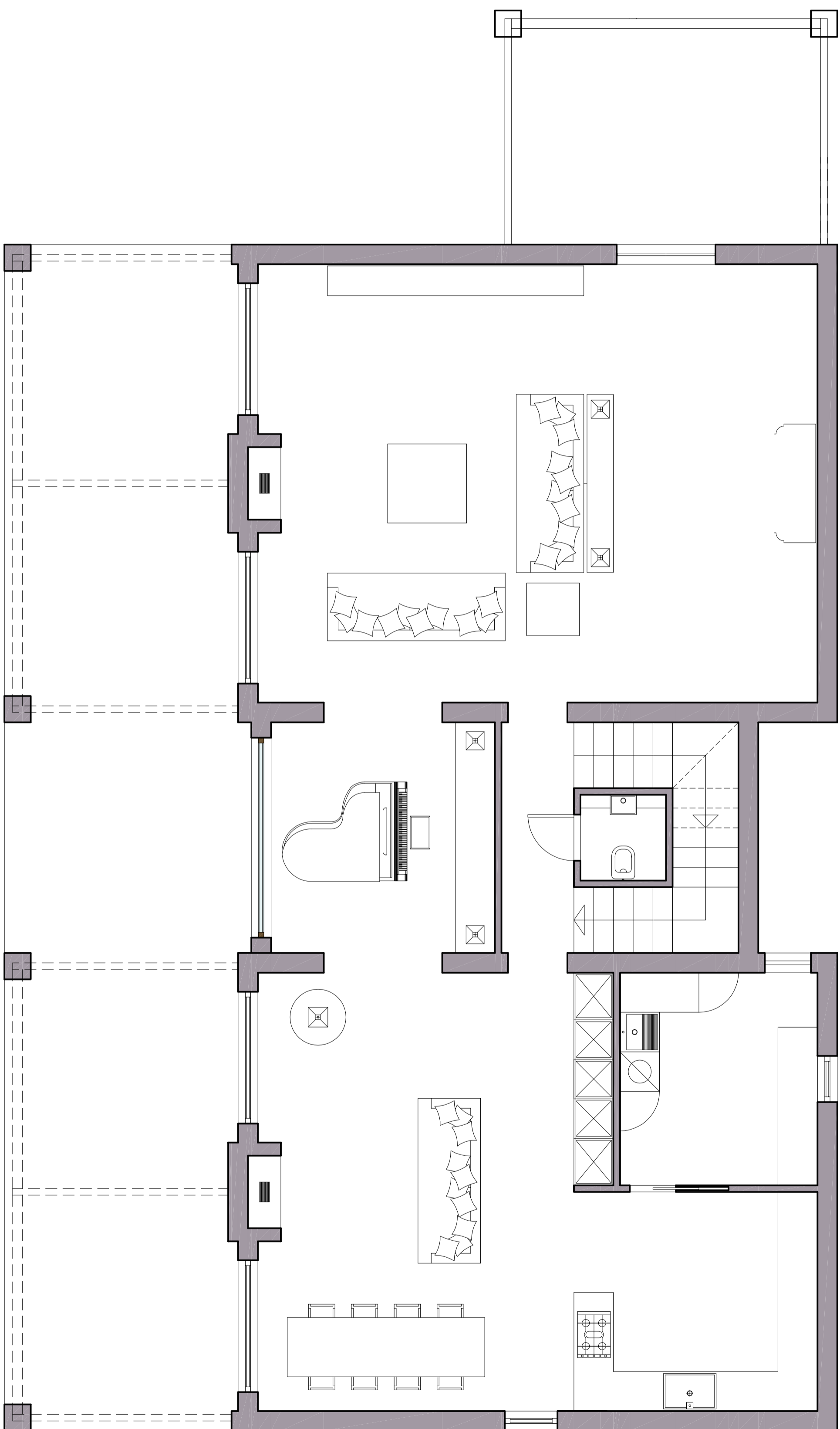
PIANTA PIANO TERRA - scala 1:50
